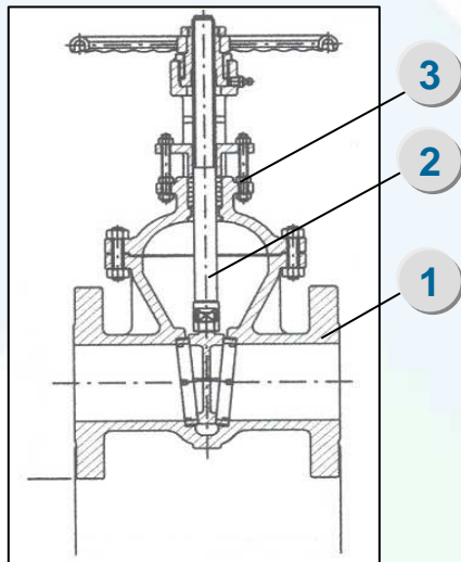
Exemplo de Válvula Gaveta
